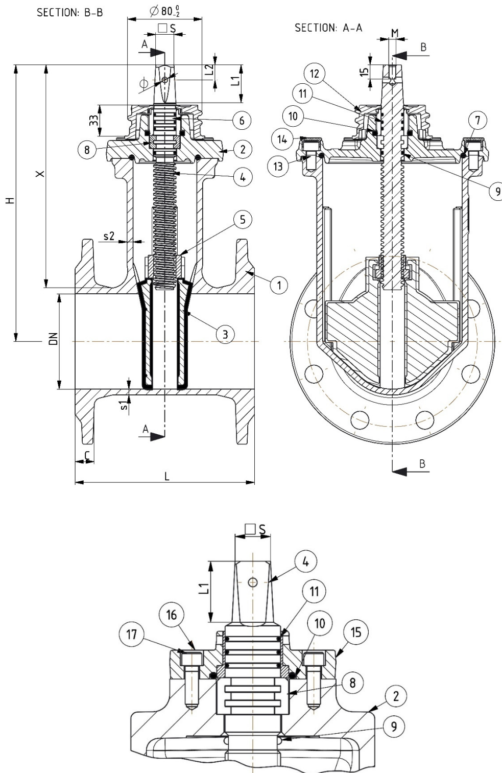
Oberes Teil von Oval-Keilschieber Haube DN 250 mm bis DN 600 mm
